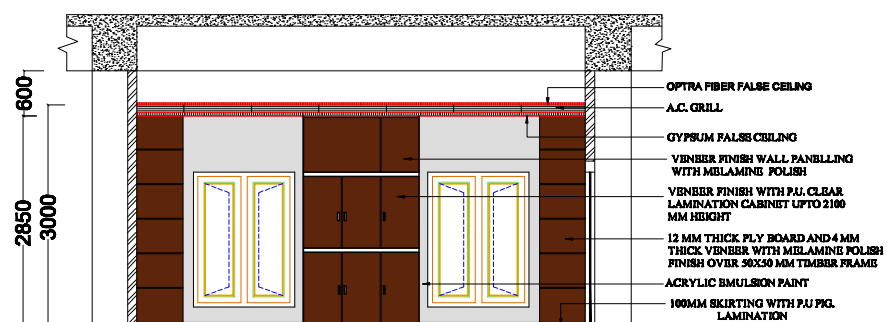
ELEVATION A
