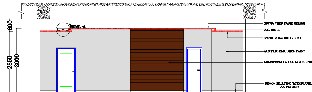
ELEVATION B
